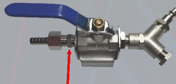
PV264B Raccord conique 1/4M 1/4M
